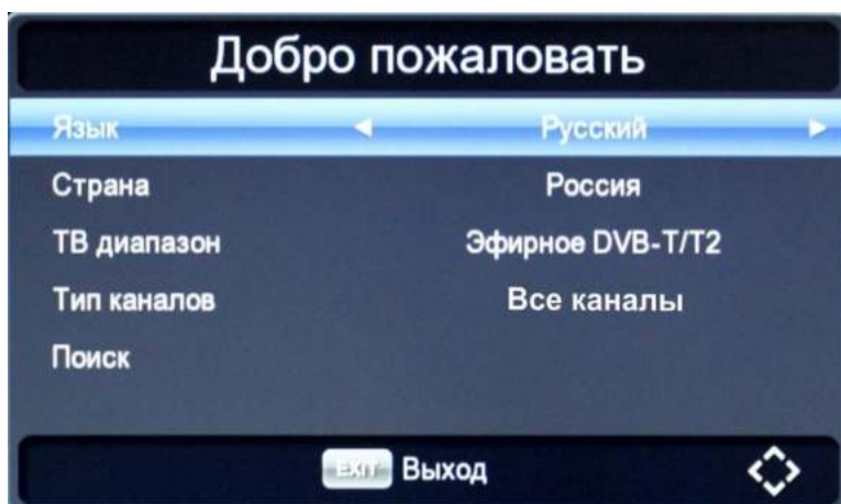
Начальное меню
