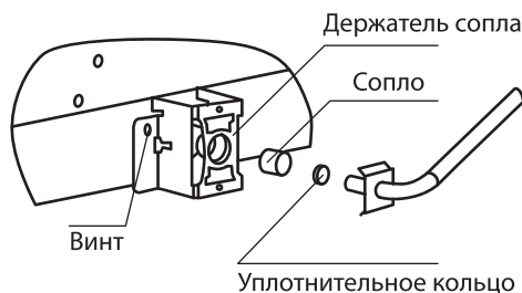
Рис. 7 Замена сопла подовой горелки
