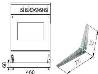
Рис. 3 Крепление плиты к стене
