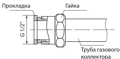
Рис. 1 Конструкция газопровода плиты
